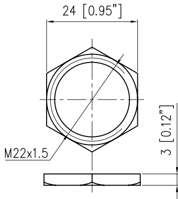
NUT M22x1.5
