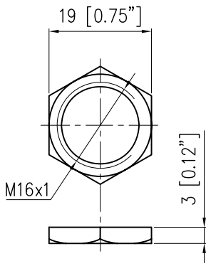
NUT M16x1
