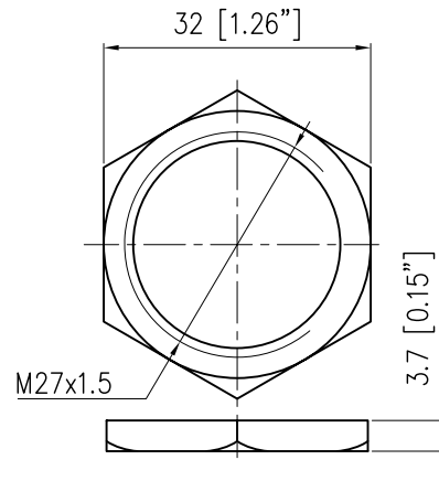
NUT M27x1.5
