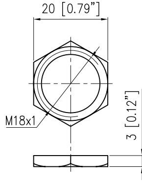
NUT M18x1
